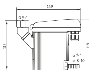
BEKOMAT® 31
