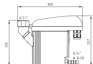
BEKOMAT® 32
